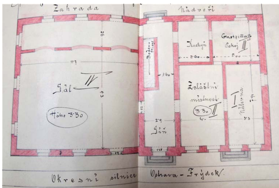
Půdorys hostince Viléma Vašíčka č. p. 44 (dnes Myslivna u kostela), r. 1912.
